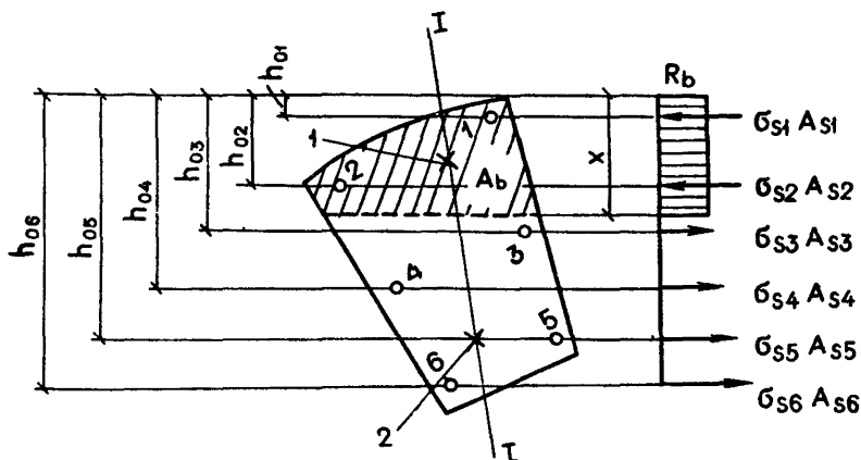
Черт. 10. Схема усилий и эпюра напряжений в сечении, нормальном к продольной оси железобетонного элемента, в общем случае расчета по прочности I-I — плоскость, параллельная плоскости действия изгибающего момента; 1 — точка приложения равнодействующих усилий в сжатой арматуре и в бетоне сжатой зоны; 2 — точка приложения равнодействующей усилий в растянутой арматуре
