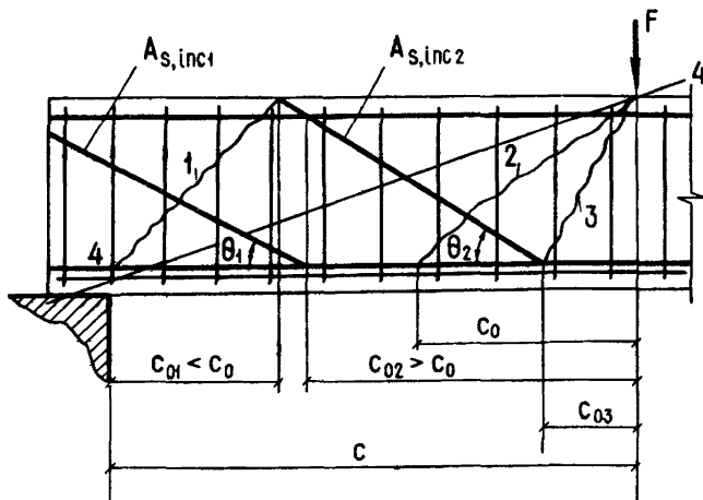
Черт. 16. К определению наиболее опасной наклонной трещины для элементов с отгибами 1, 2, 3 – возможные наклонные трещины; 4-4 – рассматриваемое наклонное сечение
