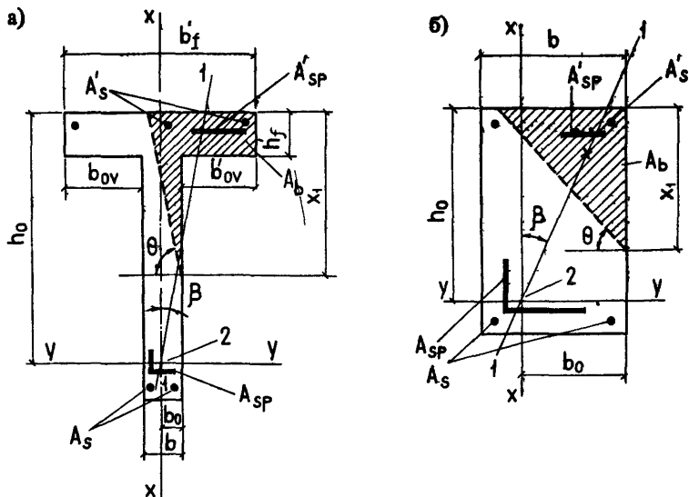
Черт. 7. Форма сжатой зоны в поперечном сечении железобетонного элемента, работающего на косоу изгиб
