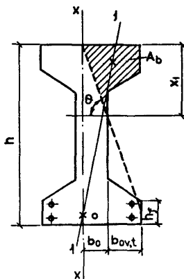
Черт. 8. Двутавровое сечение со сжатой зоной, заходящей в наименее растянутый свес полки l-l – плоскость действия изгибающего момента
