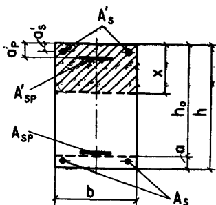
Черт. 5. Поперечное прямоугольное сечение изгибаемого железобетонного элемента
