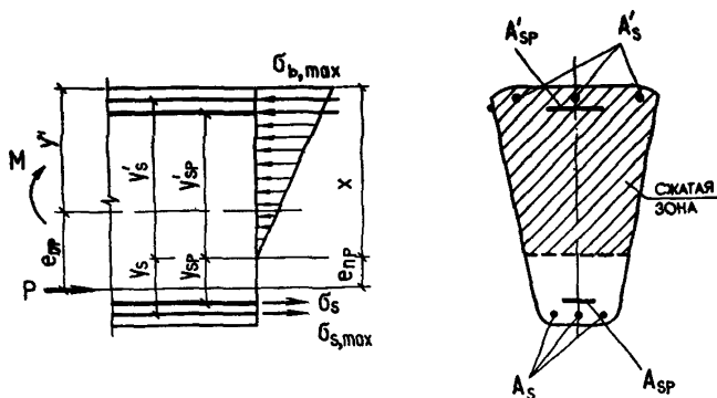
Черт. 35. Схема расположения усилей в поперечном сечении с трещиной, рассчитываемом на выносливость
