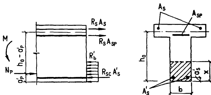
Черт. 29. Схема усилий в поперечном сечении в偏心ренно обжатого железобетонного элемента с прямоугольной сжатой зоной
