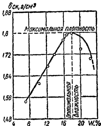
РИС. 3. КРИВАЯ ОПРЕДЕЛЕНИЯ ОПТИМАЛЬНОЙ ВЛАЖНОСТИ И МАКСИМАЛЬНОЙ ПЛОТНОСТИ ГРУНТА И ЦЕМЕНТО-ГРУНТА
