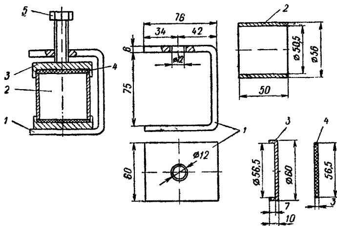
РИС. 12 ОБОЙМА ДЛЯ ПРОГРЕВА ЦЕМЕНТОГРУНТОВЫХ ОБРАЗЦОВ 1 — струбина; 2 — кольцо; 3 — крышка; 4 — резиновая прокладка; 5 — болт
