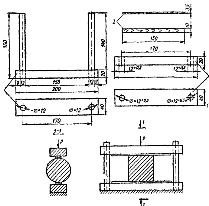
РИС. 11. ПРИСПОСОБЛЕНИЕ И СХЕМА ИСПЫТАНИЙ ОБРАЗЦОВ-ЦИЛИНДРОВ НА РАСКОЛ
