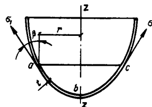
Рис. 17. Схема оболочки вращения
