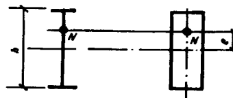
Рис. 16*. Схема внецентренно-сжатых элементов двутаврового и корабчатого сечений
