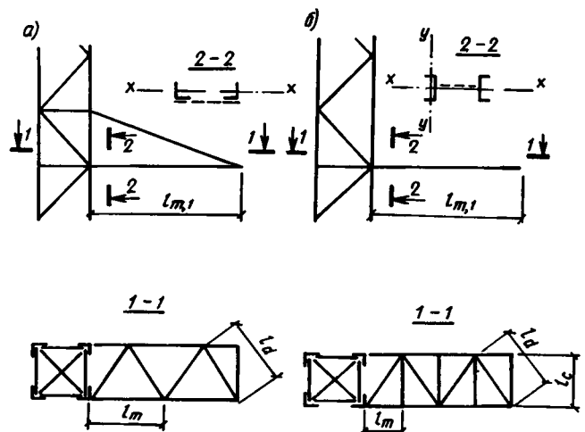
Рис. 21. Схемы траверс
