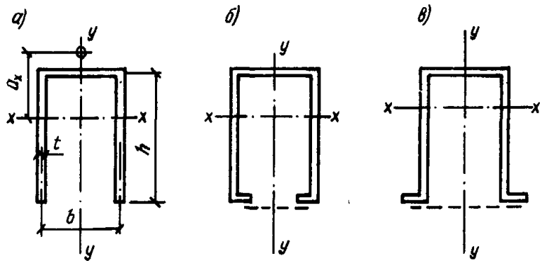
Рис. 1. П-образные сечения элементов а — открытое; б, в — укрепленные планками или решеткой
