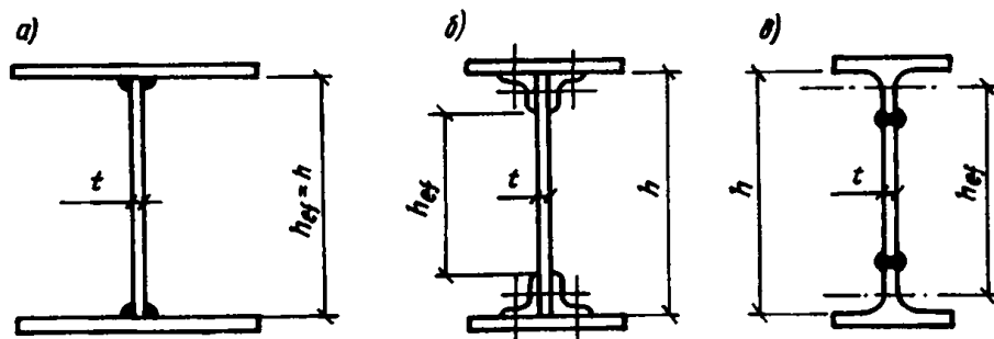
Рис. 10. Расчетная высота стенки составной балки а — сварной из листов; б — на высокопрочных болтах; в — сварной с таврами
