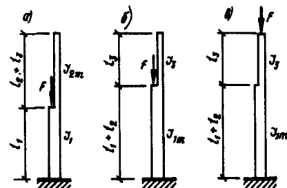
Рис. 26. Схемы одноступенчатых колонн (к табл. 71)
