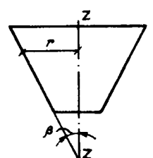
Рис. 18. Схема конической оболочки вращения
