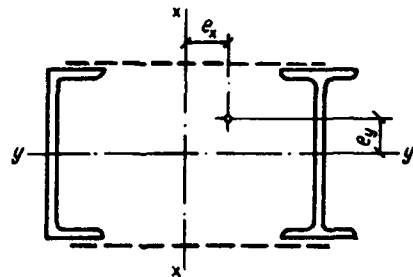
Рис. 6. Сквозное сечение стержня из двух сплошнотенчатых ветвей
