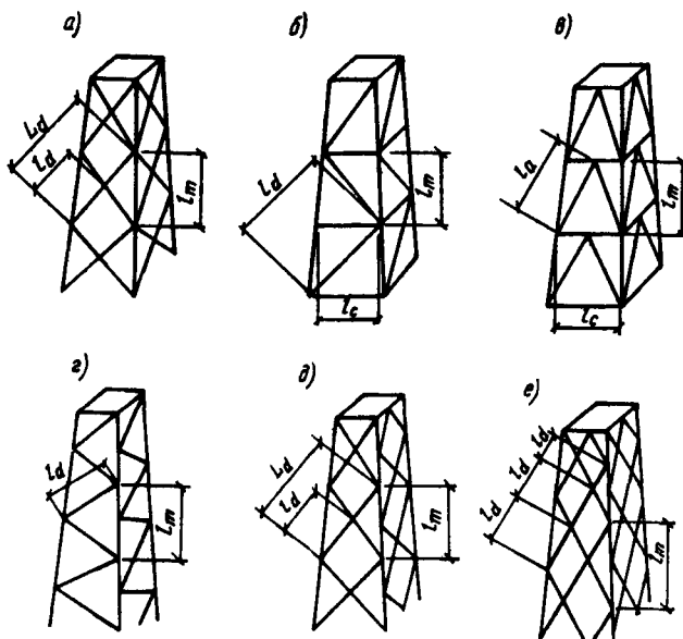
Рис. 9*. Схемы пространственных решетчатых конструкций а, б, в — с совмещенными в смежных гранях узлами; г, д, е — с несомещенными в смежных гранях узлами
