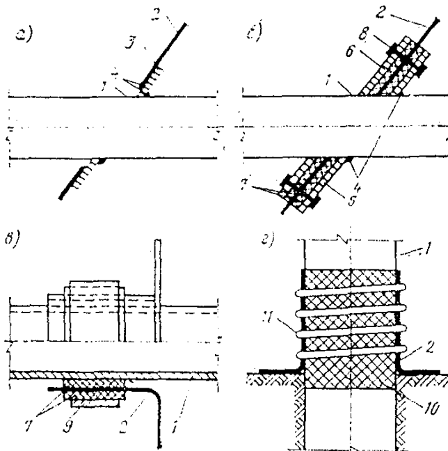
Рис. 8. Варианты сопряжения пленочного элемента с трубой
