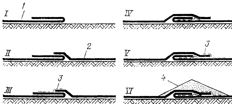
Рис. 9. Конструкция шва с использованием липкой полиэтиленовой ленты I—VI этапы производства работ; 1— край первого пленочного полотнища; 2— край второго полотнища; 3— липкая полиэтиленовая лента; 4— защитный слой грунта
