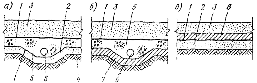
Рис. 3. Конструкции двухслойного (а, б) и комбинированного (в) противofильтрационного устройства из полиэтиленовой пленки
