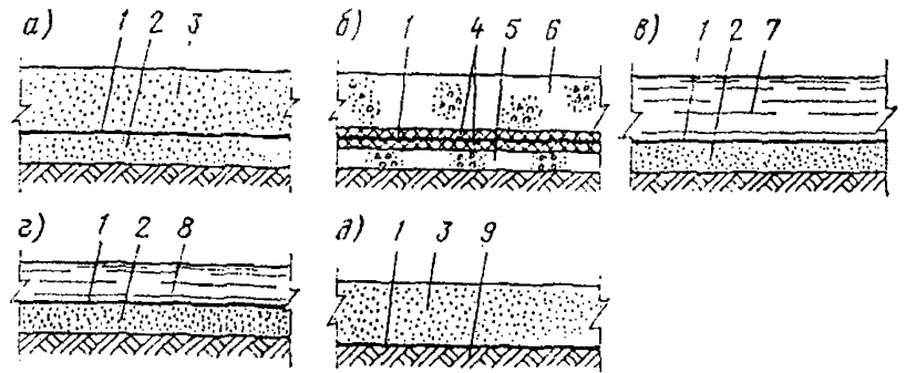
Рис. 2. Варианты конструкций однослойного противofильтрационного устройства из полиэтиленовой пленки
