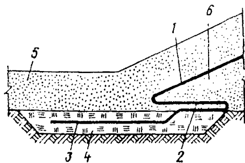
Рис. 2. Вариант конструкции узла сопряжения пленочного элемента с уширенной штрабой 1 — полиэтиленовая пленка; 2 — компенсирующая складка; 3 — заделанный край полиэтиленовой пленки; 4 — пластичный грунт, заполняющий уширенную штрабу; 5 — защитный слой из песка; 6 — подстилающий слой из песка
