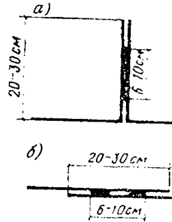
Рис. 8. Двойные сварные швы а — Т-образный; б — нахлесточный
