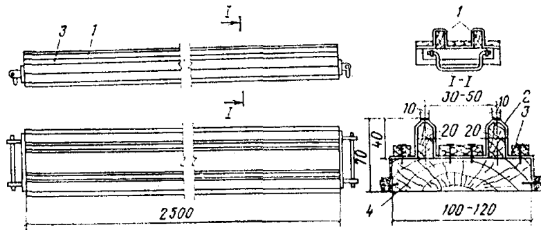
Рис. 2. Схема сварочной рейки
