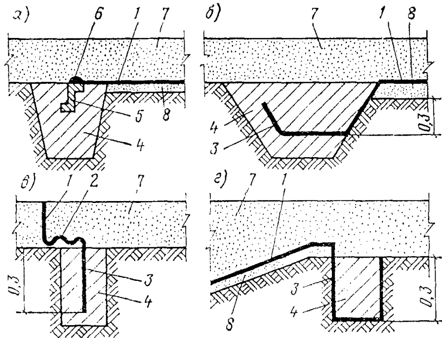
Рис. 1. Варианты конструкций узлов сопряжения пленочного противодиффузионного устройства с зубом (а, б) и глубокой штрабой (в, г) 1 — полиэтиленовая пленка; 2 — компенсирующая складка, 3 — заделанный край пленочного элемента; 4 — пластичный грунт (бегон), заполняющий штрабу (зуб); 5 — профиль из пластмассы, 6 — сварной шов, 7 — защитный слой из песка; 8 — подстилающий слой из песка
