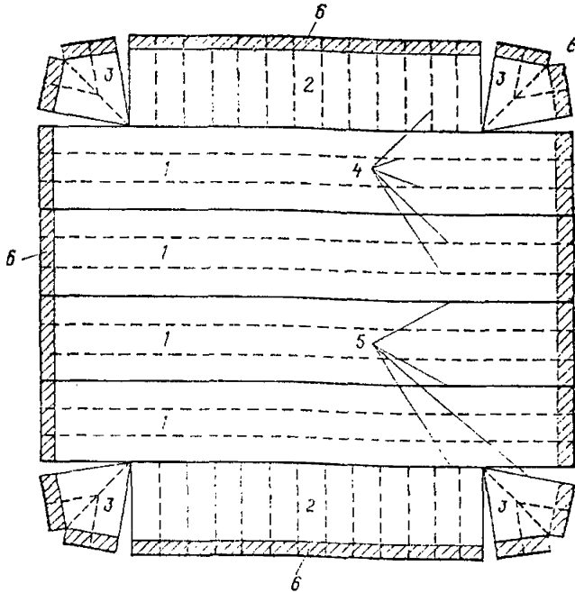
Рис. 6. Вариант размещения полотнищ на карте экранирования 1 — основное полотнище; 2 — боковое полотнище; 3 — угловое полотнище; 4 — швы сварки в цехе; 5 — монтажные швы; 6 — часть экрана, заделываемая в траншею на гребне дамбы
