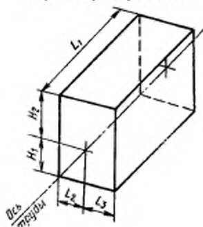
Габаритные размеры счетчиков
