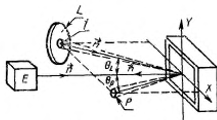
1 — проекция апертуры для приема света на отражающую поверхность источника, используемого при измерении; E — источник света; P — фотометр
