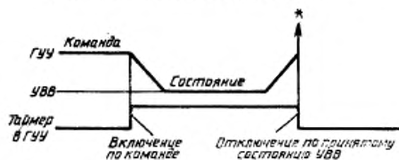
Временная диаграмма для команд управления
