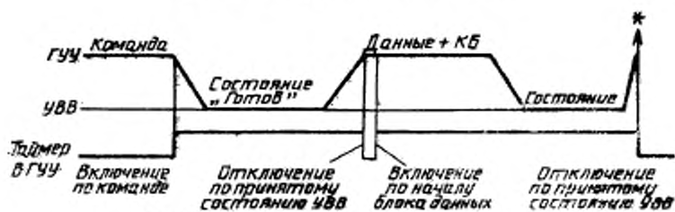
Временная диаграмма для команд записи
