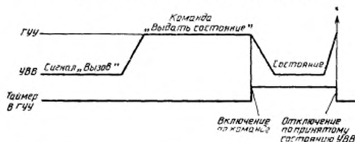
Временная диаграмма обработки сигнала «Вызов»
