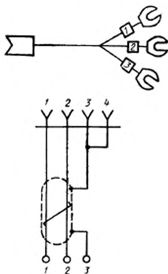
Схема распайки кабеля
