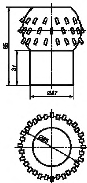
Защитный колпачок
