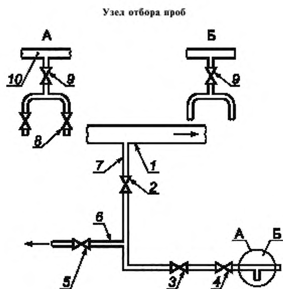
А — узел отбора проб с использованием пробоотборной пробирки (черт. 5); Б — узел отбора проб с использованием пробоотборной пробирки (черт. 4); 1 — трубопровод для сжиженного безводного аммиака; 2, 3, 8, 9 — вентили для подачи сжиженного безводного аммиака; 4 — вентиль тонкой регулировки; 5 — вентиль для сброса аммиака в дренажную систему; 6 — продувочная линия; 7, 10 — пробоотборная линия
