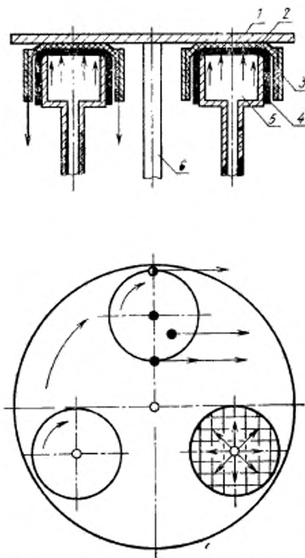
1 — истирающий диск; 2 — проба; 3 — обойма; 4 — мембрана; 5 — головка; 6 — ось
