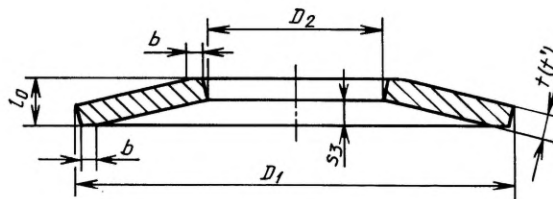
Пружина типа 2
