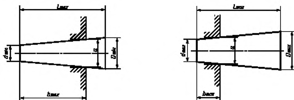
Рисунок А.3 — Изменение глубины проникновения b у конусообразных испытательных шупов
