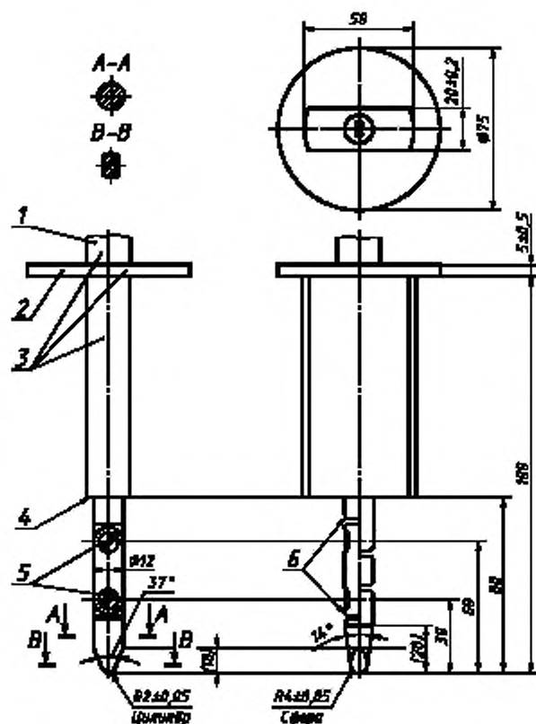
Рисунок 1 — Испытательный щуп А
