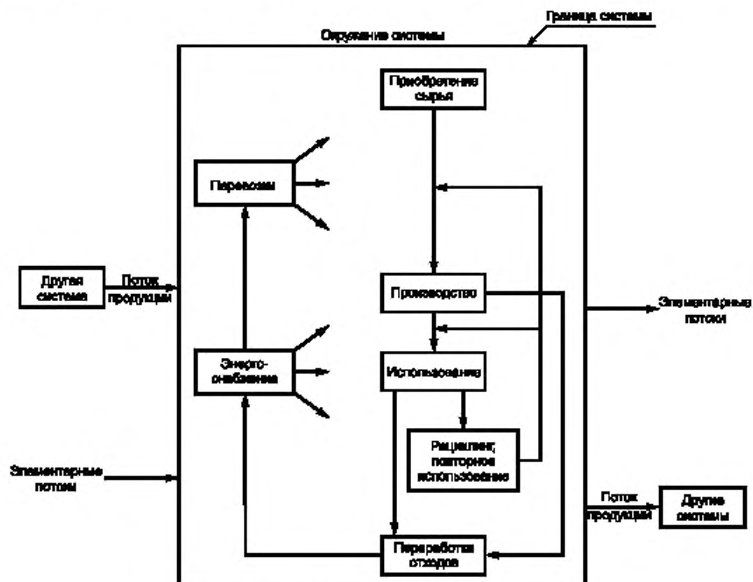
Рисунок 1 — Пример производственной системы
