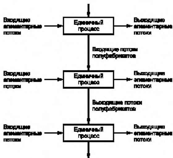
Рисунок 2 — Пример совокупности единичных процессов в производственной системе
