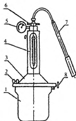
Рисунок 5 — Поромер
