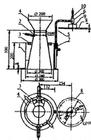
Рисунок 2 — Установка типа Вебе
