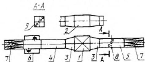
Испытательный стенд для измерения статического снижения шума глушителем внутри воздуховода методом с замещающим воздухопроводом
