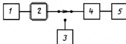
1 — низкочастотный генератор сигналов; 2 — передатчик; 3 — высокока частотный ваттметр; 4 — эквивалент антенны; 5 — высокока частотный вольтметр
