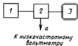
1 — генератор модулирующего сигнала (сигналов); 2 — низкочастотное согласующее переходное устройство 1-го типа; 3 — передатчик
