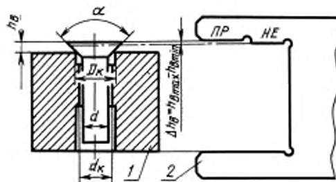
1 — ступка калибра; 2 — скоба калибра или индикатор
