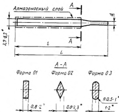
Тип 1. Прямые одноконцевые надфили Исполнение 1. Тулоносые надфили
