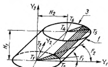
Черт. 3
