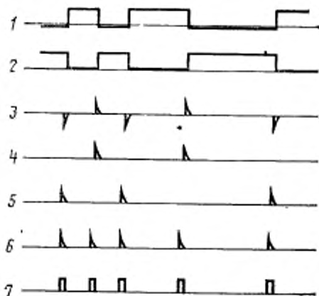
1—входной сигнал; 2—сигнал после формирователя; 3—сигнал на выходе дифференцирующей цепи; 4—неинвертируемые положительные импульсы; 5—сигнал на выходе мультивибратора; 6—сигнал на входе мультивибратора; 7—выходные импульсы
