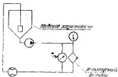
Схема стенда для испытания на прочность
