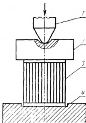
1—гризевой шток; 2—гризевая шайба; 3— фильтроэлемент; 4—основание
