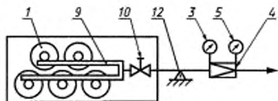
г) Рампа с баллонами, соединенными в группу
