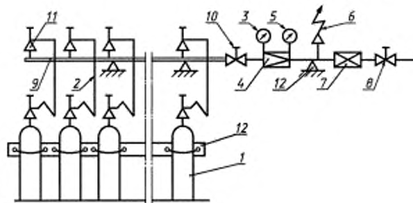
г) Рампа с баллонами, соединенными в группу
