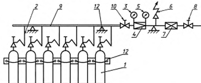
в) Рампа с более 6 баллонами
