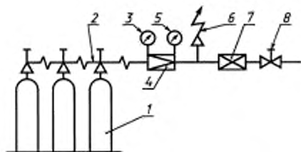
б) Рампа с 6 и менее баллонами
