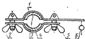
1 — верхняя половина дуги; 2, 5 — гайки бо- ранныхые; 3 — вкладыши; 4 — нижняя половина ду- ги; 6 — динамометр или груз
