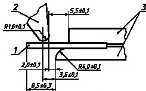
Детали и размеры кромки и зажимного устройства (размещение испытуемого образца без надреза)
