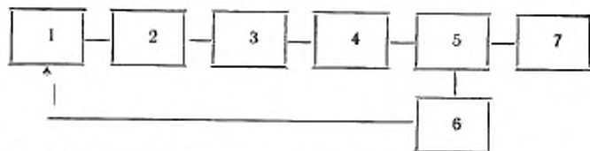
1—генератор СВЧ; 2—развязывающий аттенюатор или ферритовый вентиль; 3—регулируемый аттенюатор; 4—поверяемый ваттметр; 5—измерительная линия; 6—компаратор импульсной мощности; 7—подвижный короткозамыкатель
