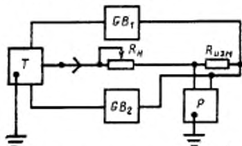
Т—телеграфный аппарат; GB_1 , GB_2 —линейные батареи; R_{н} —сопротивление нагрузки; R_{изм} —измерительное сопротивление; P —измерительный прибор
