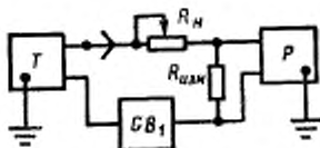
Т—телеграфный аппарат; GB_1 —линейная батарея; R_{н} —сопротивление нагрузки; R_{изм} —измерительное сопротивление; P —измерительный прибор
