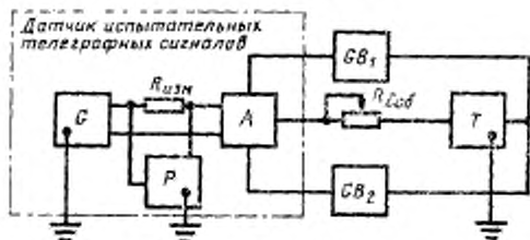
G—генератор прямоугольных импульсов; R_{изм} —измерительное сопротивление; P—измеритель временных интервалов; A—выходное реле; GB_1 , GB_2 —линейные батареи; R_{доб} —добавочное сопротивление; T—телеграфный аппарат
