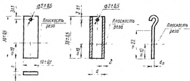
Образец из проволоки
