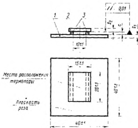
1—нижняя пластина; 2—верхняя пластина; 3—прокладка
