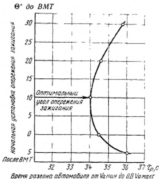
Динамическая характеристика автомобиля по углу опережения зажигания при разгоне
