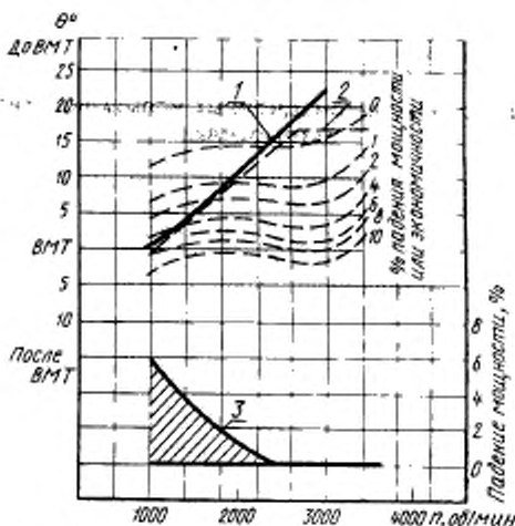
1 детонационная характеристика заданного бензина; 2 выбранная характеристика автомата; 3 потери мощности
