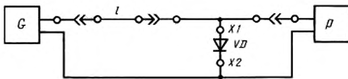
G — генератор импульсов; l — развязывающий кабель; P — измерительное устройство; X1 и X2 — контакты подключения; VD — проверяемый диод
