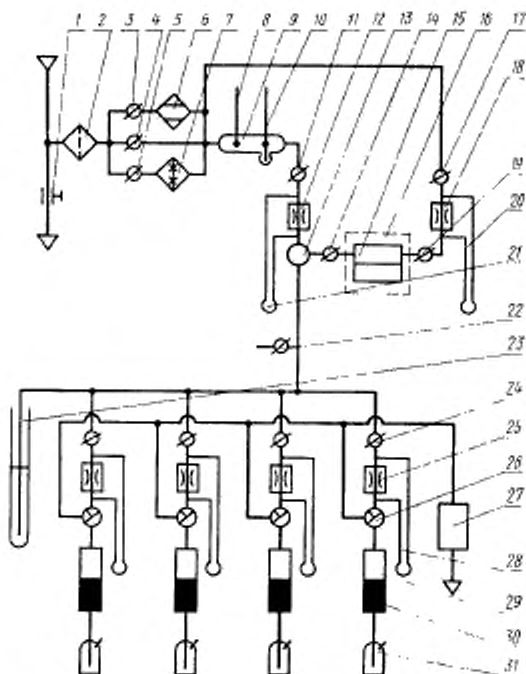
Схема динамического прибора
