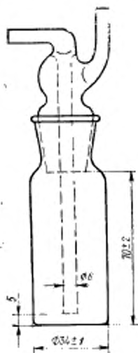
Индикаторная склянка
