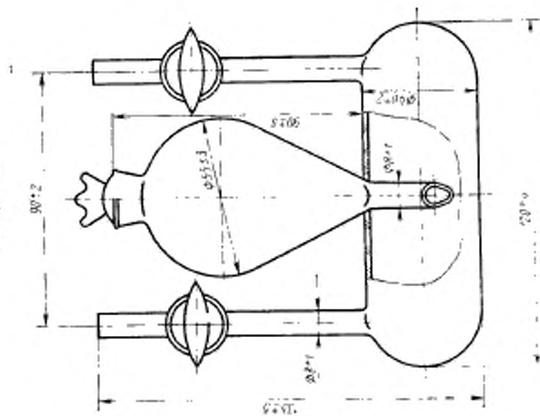
Испаритель
