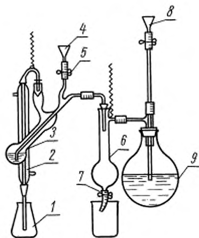
Черт. 2
