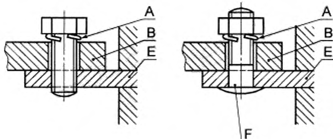
A — запирающее устройство; B — кабельный наконечник или шина; E — неподвижная часть; F — штырь
