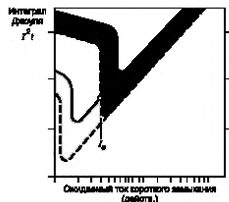
Рисунок F.3 — АВО с теплоэлектромагнитным расцепителем, резервной защитой, осуществляемой автоматическим выключателем с теплоэлектромагнитным расцепителем
