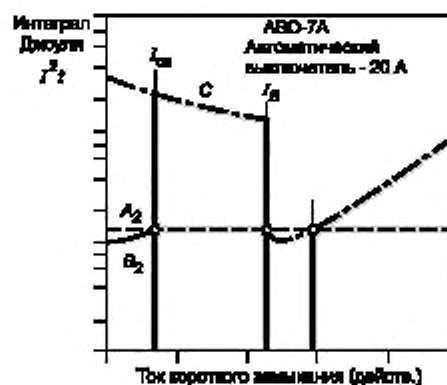
Рисунок F.8 — Примеры подлинной и ошибочной координации
