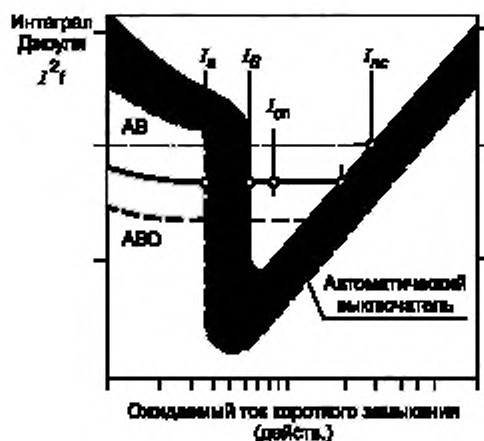
Рисунок Е.1 — АВО с тепловым расцепителем, резервной защитой, осуществляемой автоматическим выключателем с теплоэлектромагнитным расцепителем
