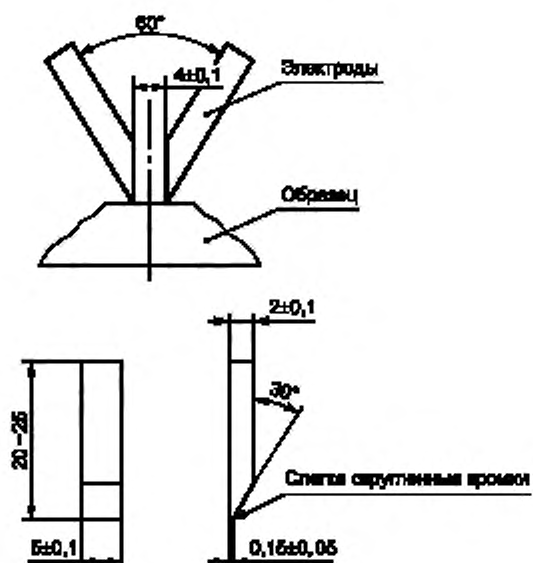
Рисунок 9 — Монтаж и размеры электродов для испытания на трекинговость
