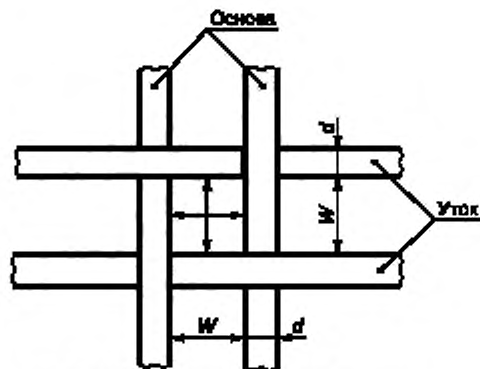
Рисунок 1 — Ячейка сетки
