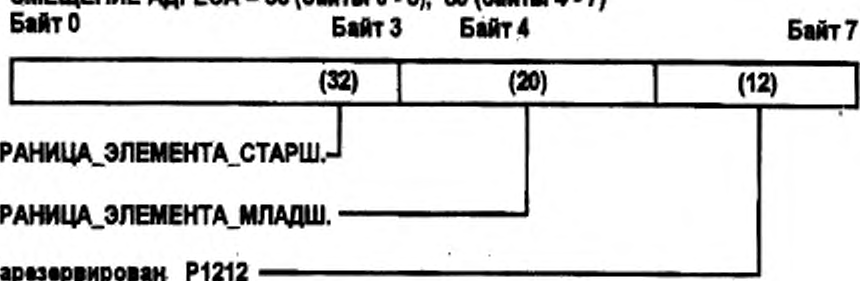
Рисунок 3-15 — Формат данных РУСа ГРАНИЦА_ЭЛЕМЕНТОВ
