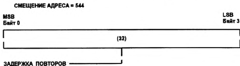
Т а б л и ц а 3—43 — Описание разрядов регистра ЗАДЕРЖКА_ПОВТОРОВ_ПРИ_ЗАНЯТОСТИ
