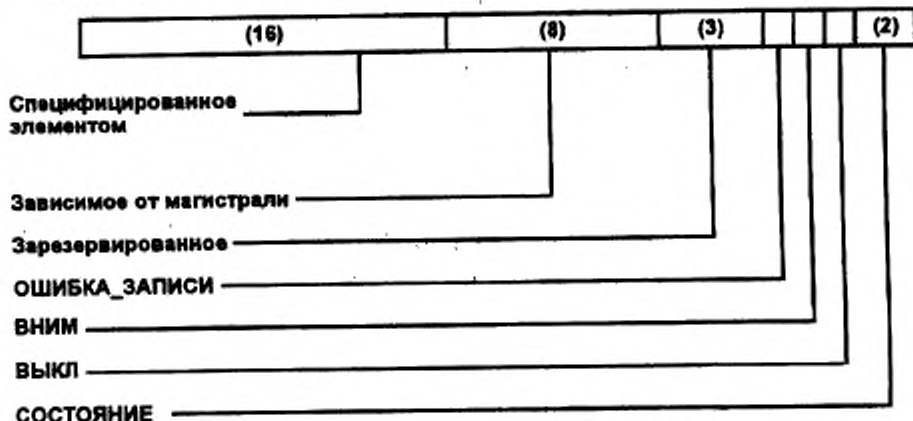
Рисунок 3-5 — Поля в РУСх ОЧИСТКА_СОСТОЯНИЯ и УСТАНОВКА_СОСТОЯНИЯ, используемые в ФБ+.
