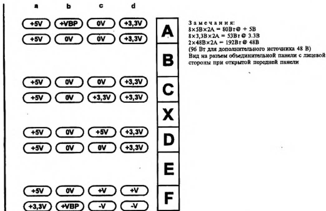
Рисунок 7—16 — Распределение контактов питания для разъемов профиля Б
