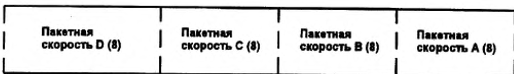
Рисунок 3—31 — Формат РУС СКОРОСТЬ_ПАКЕТА
