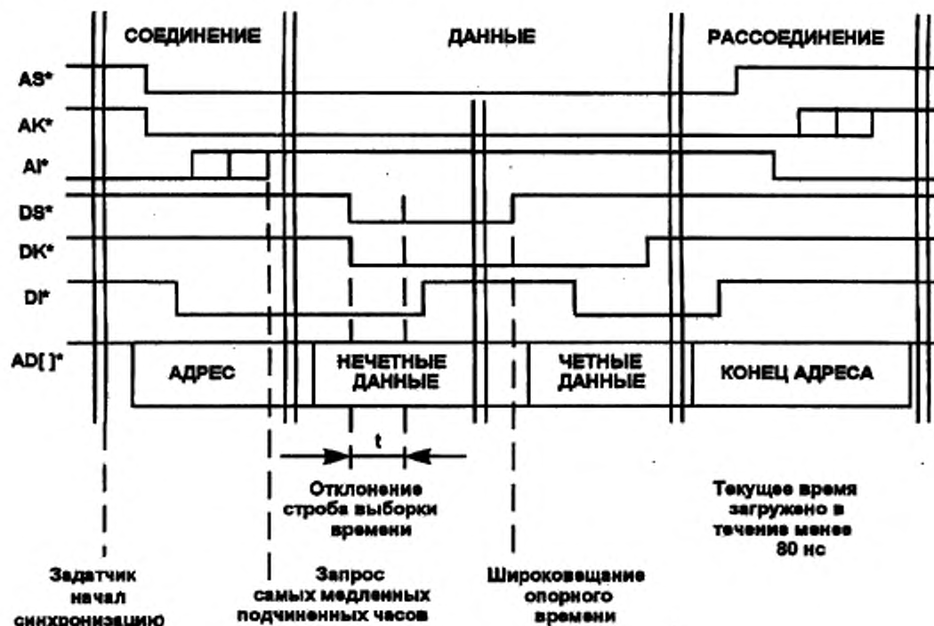
Рисунок 3—4 — Синхронизация часов
