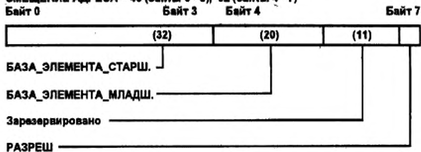
Рисунок 3-14 — Формат данных РУСа БАЗА_ЭЛЕМЕНТОВ
