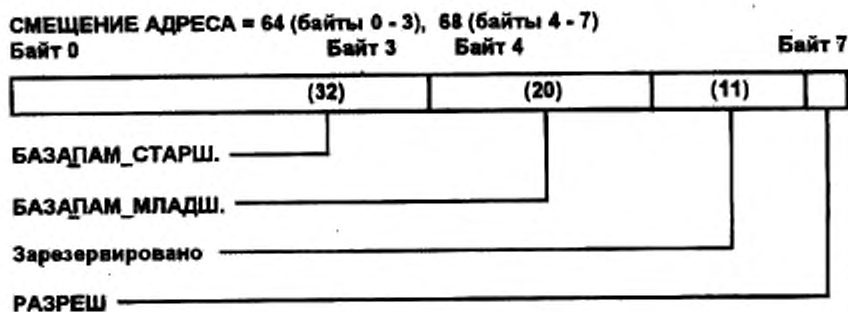
Рисунок 3—16 — Формат данных РУС БАЗА_ПАМЯТИ
