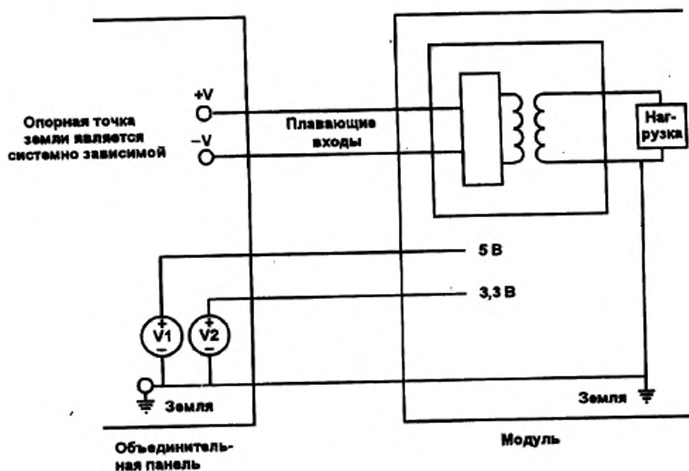
Рисунок 7-1 — Шины питания Профиля Б
