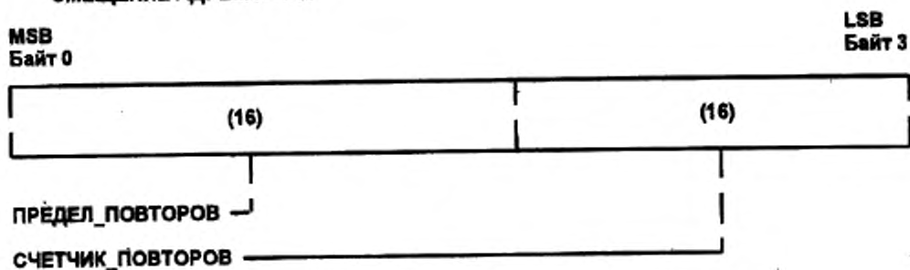
Рисунок 3-26 — Регистр СЧЕТЧИК_ПОВТОРОВ_ПРИ_ОШИБКЕ
