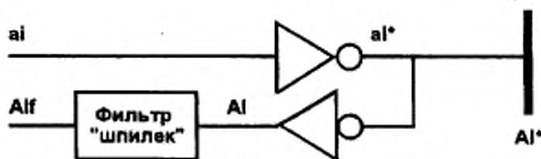
Рисунок 2.1 — Соглашения о сигналах
