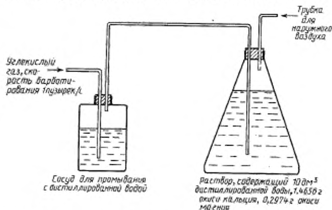
Рисунок 1 — Схема аппарата для приготовления воды с искусственной жесткостью
