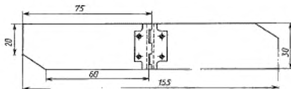
Рисунок 2 — Давящая пластинка
