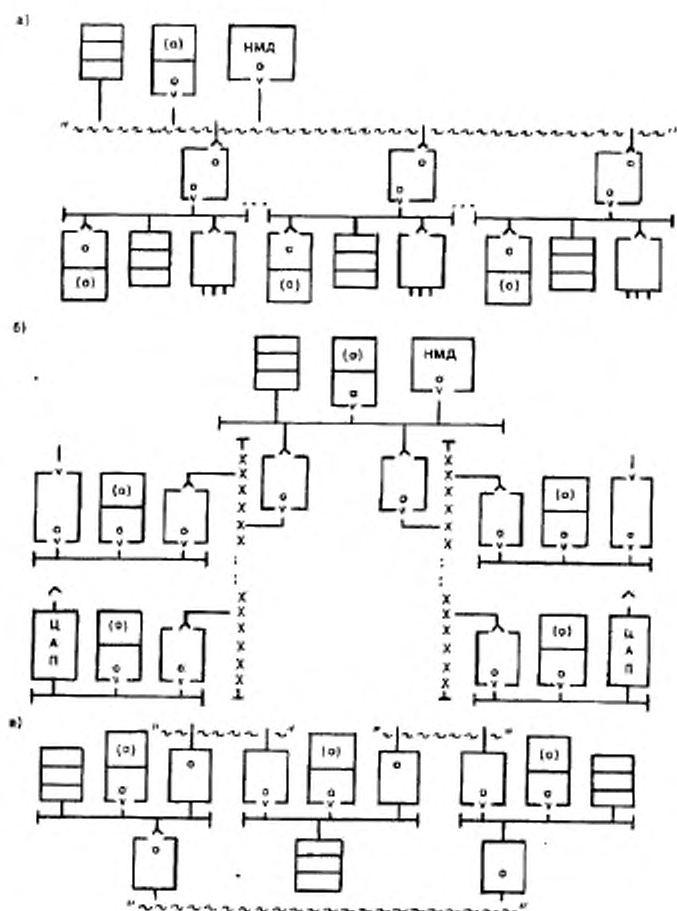
а) трехуровневая линейная структура на основе кабельной межконтурной магистрали; б) трехуровневая древовидная структура; в) кольцевая структура
