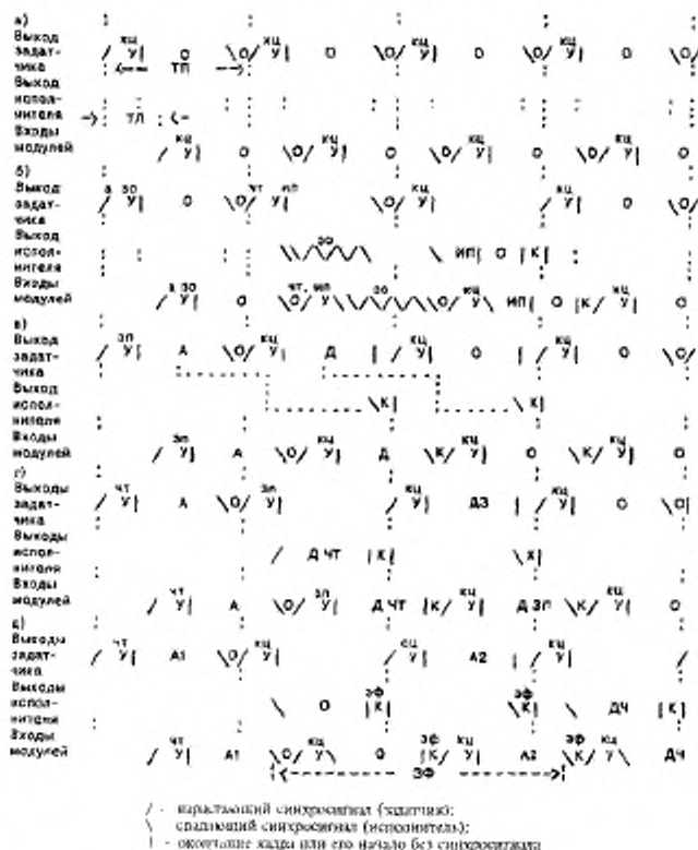
а) свободная магистраль; б) двукратная приоритетная 30; в) единичный индекс члена данных; г) единичный индекс члена данных; д) индекс члена данных с кадровой фазой передачи
