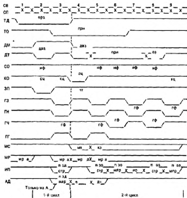
Рисунок Б.1 — Временные диаграммы циклов арбитража
