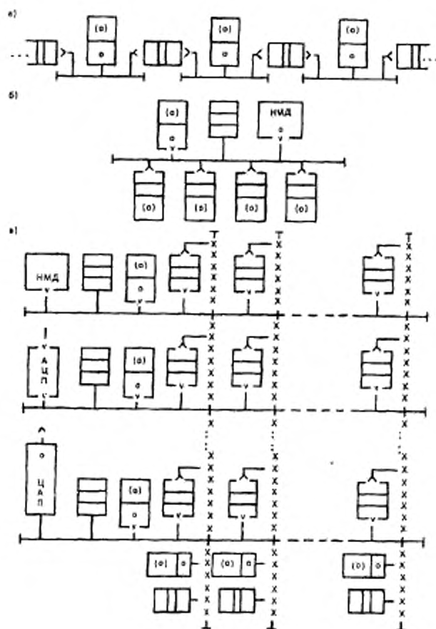
а) система последовательной обработки данных со связями через двухсторонние ОЗУ; б) система параллельной обработки; в) матричная структура на основе двухсторонних ОЗУ
