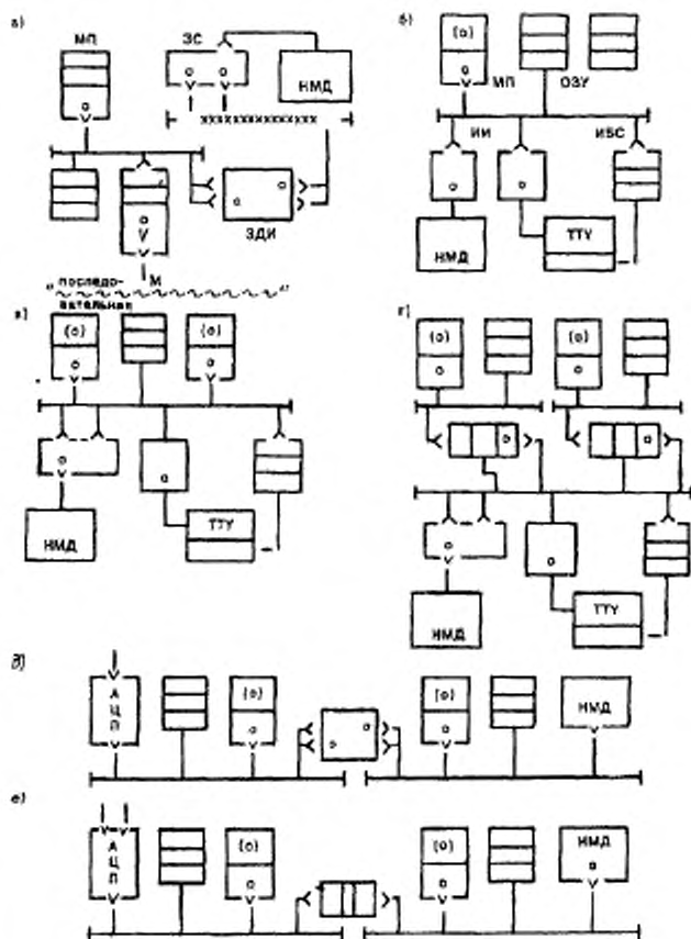
а) однопроцессорный микроЭВМ, подключение через кабельную матрицу МСИ к НМД; б) персональный ЭВМ ТТУ; в) двухпроцессорный микроЭВМ; г) вычислительная система с локальными подсистемами обработки данных; д) связь двух микроЭВМ через ЗДИ (прямой доступ в память); е) связь двух микроЭВМ через ИС (общее ОЗУ).
