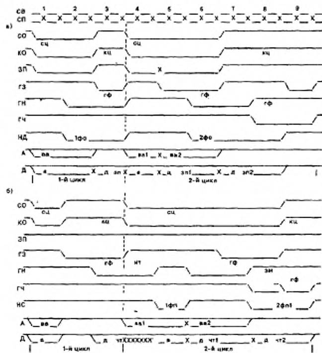
а) медленный датчик (1-й цикл), медленный исполнитель (2-й цикл)-б) медленный датчик (1-й цикл), медленный датчик (2-й цикл)
