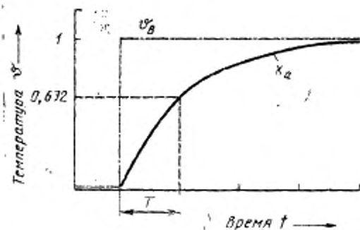
Рисунок ВВ1 — Определение постоянной времени методом быстрого изменения температуры
