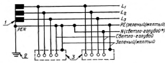
1 — точка заземления энергосистемы; 2 — земля; 3 — открытые проводящие части; L_1, L_2, L_3 — фазные проводники энергосистемы; N — нулевой проводник; PE — защитный проводник
