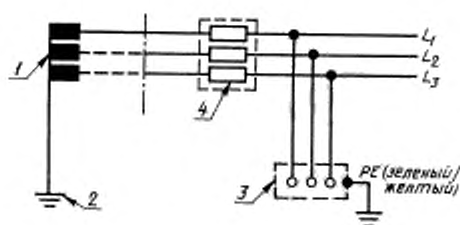
1 — точка заземления энергосистемы; 2 — земля; 3 — открытые проводящие части; 4 — реактор ограничения тока нулевой последовательности; L_1 , L_2 , L_3 — фазные проводники энергосистемы; PE — защитный проводник
