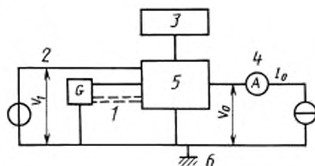
G — источник напряжения и генератор импульсов; I — другие входы; 2 — измеряемый вход; 3 — источник питания; 4 — измеряемый выход; 5 — измеряемая схема; 6 — опорная шина
