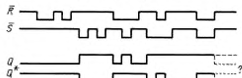
Временная диаграмма
