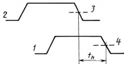
Время удержания (типовые формы сигнала)
