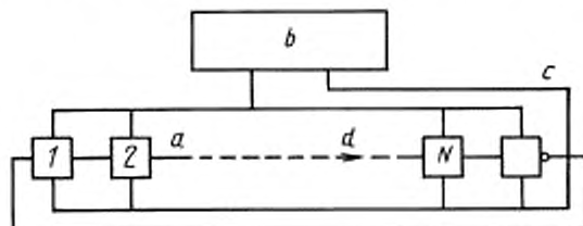
Кольцевой генератор для неинвертирующих N-схем
