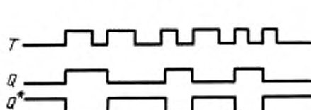
Временная диаграмма
