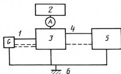
G — источник напряжения и генератор импульсов; 1 — вход(ы); 2 — источник питания; З — измеряемая схема; 4 — выход(ы); 5 — цепь на выходе; 6 — опорная шина
