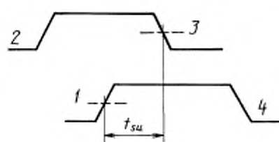
Время установления (типовые формы сигнала)
