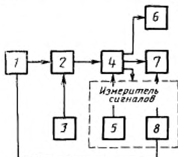
1 — оптическая система, 2 — передающая трубка, 3 — генератор разверток; 4 — видеосигналы; 5 — генератор калибровочных прямоугольных импульсов (ГКИ); 6 — видеоконтрольное устройство (ВКУ); 7 — осциллограф выделения строки (ОВС); 8 — устройство управления световым затвором
