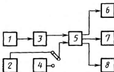
1 — оптическая система; 2 — генератор калиброванных прямоугольных импульсов (ГКИ); 3 — передающая трубка; 4 — генератор калиброванных сигналов; 5 — видеоусилитель; 6 — видео-контрольное устройство (ВКУ); 7 — осциллограф выделения строки (ОВС); 8 — измеритель шумов
