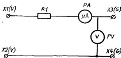
X1(V), X2(V) — выводы для подключения электродов трубки; R1 — ограничительный резистор; PA — микроамперметр; PV — вольтметр; X3(G), X4(G) — выводы для подключения источника питания
