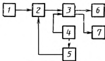
1 — оптическая система; 2 — передающая трубка; 3 — видеоусилитель; 4 — генератор калиброванных импульсов (ГКИ); 5 — формирователь запирающих импульсов; 6 — видеоконтрольное устройство (ВКУ); 7 — осциллограф выделения строки (ОВС)
