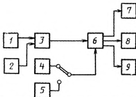
1 — основная оптическая система; 2 — дополнительная оптическая система; 3 — передающая трубка; 4 — генератор калибровочных прямоугольных импульсов (ГКИ); 5 — генератор калибровочных сигналов; 6 — видеоусилитель; 7 — видеоконтрольное устройство (ВКУ); 8 — осциллограф выделения строки (ОВС); 9 — измеритель шумов
