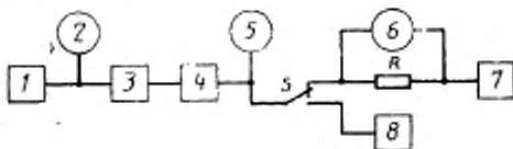
1, 7 — генераторы, 2, 5, 6 — вольтметры; 3 — согласующее звено, 4 — измеряемый усилитель; 8 — эквивалент нагрузки; S — переключатель; R — резистор, сопротивление которого равно номинальному сопротивлению нагрузки
