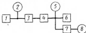
1 — генератор; 2, 5, 8 — вольтметры; 3 — согласующее звено; 4 — измеряемый усилитель; 6 — эквивалент нагрузки; 7 — фильтр
