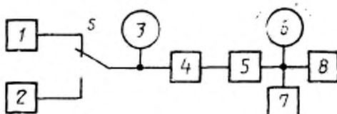
1 — генератор υψηшек тона; 2 — генератор; 3, 6 — вольтметры; 4 — согласующее звено; 5 — измерительный усилитель; 7 — самописец; 8 — эквивалент нагрузки; 5 — переключатель
