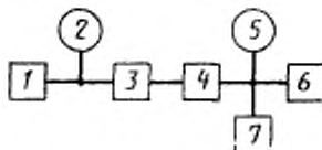
1 — генератор; 2, 5 — вольтметры; 2 — согласующее звено; 4 — измеряемый усилитель; 6 — эквивалент нагрузки; 7 — прибор для измерения гармонических искажений
