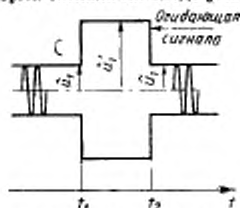
Форма сигнала на входе усилителя
