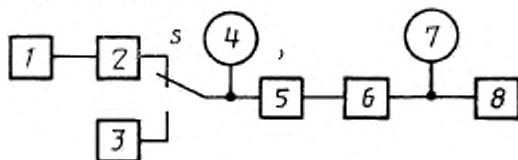
1 — генератор шумового сигнала; 2 — фильтр ФПШМ; 3 — генератор; 4 — вольтметр; 5 — согласующее звено; 6 — измеряемый усилитель; 7 — вольтметр средних квадратичных значений; 8 — эквивалент нагрузки; S — переключатель
