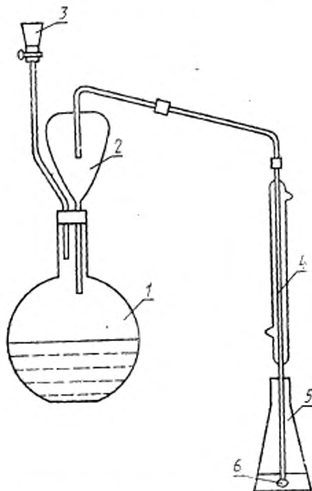
1 — реакционная колба вместимостью 250—300 см 3 ; 2 — каплеуловитель; 3 — капельная воронка с краном; 4 — холодильная трубка; 5 — приемник; 6 — барботер
