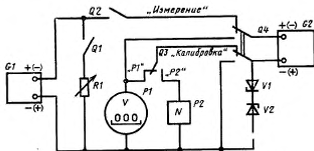
G1 —источник исследуемого постоянного напряжения (испытываемый преобразователь); G2 —источник постоянного напряжения с нестабильностью в течение времени измерения не более 0,02% и допускающий работу на противо-э.д.с.; R1 —нагрузка; Q1 , Q2 —выключатель; Q3 , Q4 —переключатель; V1 , V2 —стабилизатор типов Д816, Д817; P1 —цифровой вольтметр; P2 —регистрирующий измерительный прибор.
