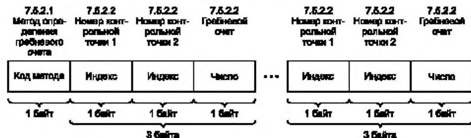
Рисунок 7 — Диаграмма формата данных гребневого счета
