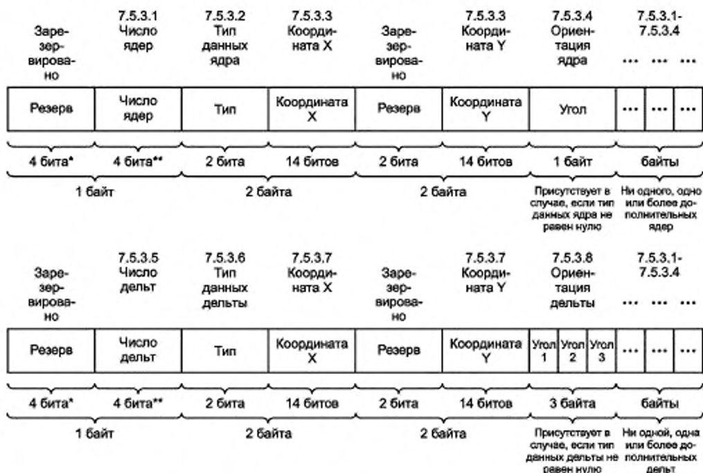
Рисунок 8 — Диаграмма формата данных ядра и дельты
