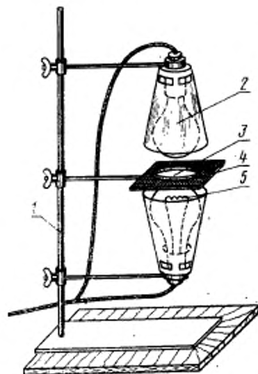
1—штатив; 2—рефлектор из жести; 3—алюминевая чашка; 4—асбестовая сетка; 5—электрическая лампа.
