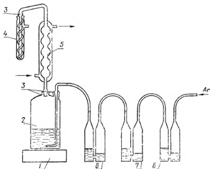
1—электролитика; 2—сосуд реакционный с восстановительной смесью; 3—шлифы; 4—приемник с щелочным раствором гидросиламина и трилона Б (спиральная кварцевая засадка, приваренная к наружной стороне выходной трубки обратного холодильника); 5—обратный холодильник; 6, 7—барботер с 25 %-ным раствором пиригаллола в 25 %-ном растворе едкого кали; 8—барботер с дистиллированной водой.
