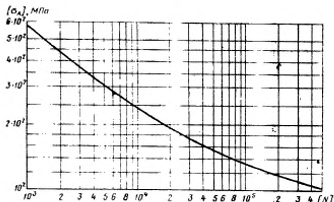
Расчетная кривая усталости для углеродистых сталей до температуры 380°C
