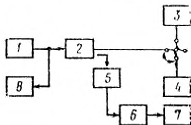
1—генератор сигналов НЧ по п. 3.2.8; 2—радиопередатчик; 3—антенна; 4—эквивалент антенны по п. 3.2.3; 5—направленный ответвитель по п. 3.2.4; 6—девиометр по п. 3.2.10; 7—измеритель нелинейных искажений по п. 3.2.11; 8—вольтметр по п. 3.2.9
