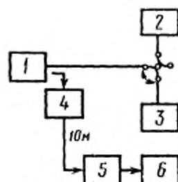
1—радиопередатчик; 2—антенна; 3—эквивалент антенны по п. 3.2.3; 4—направленный ответвитель по п. 3.2.4; 5—фильтр по п. 3.2.7; 6—селективный вольтметр по п. 3.2.12
