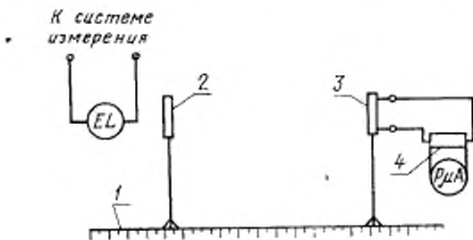
EL —источник излучения с T_{\text{н}} 2850 К; 1—фотометрическая скамья; 2—шторка; 3—фотоэлемент; РМА —прибор, измеряющий фототок (микроамперметр М95 со шкалой 10—100 мкА); 4—шунт
