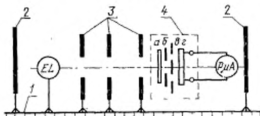
Схема фотометрической установки для измерения цветовой температуры
