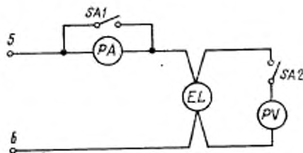
Схема системы измерения электрических параметров ламп накаливания
