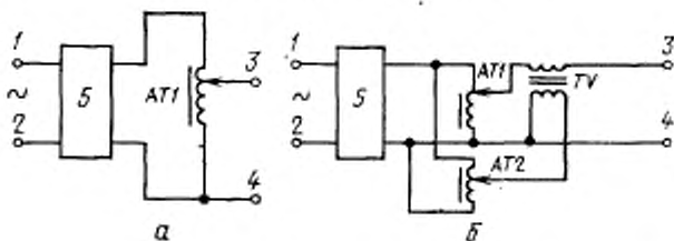
Схемы систем питания переменным током
