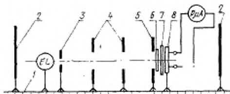
Схема фотометрической установки для измерения силы света
