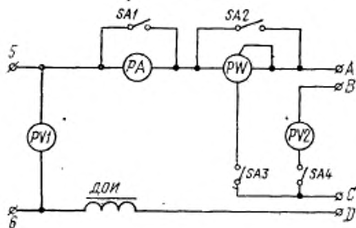
Схема системы измерения электрических параметров разрядных ламп
