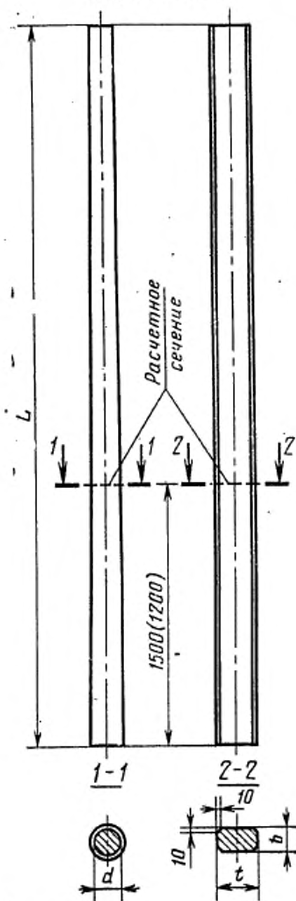
Опора типа 1
