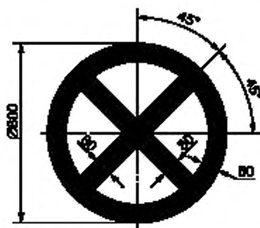
Рисунок 2 — Условное обозначение подруливающего устройства
