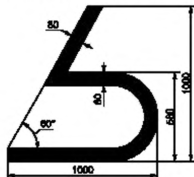
Рисунок 1 — Условное обозначение бульбообразного носа
